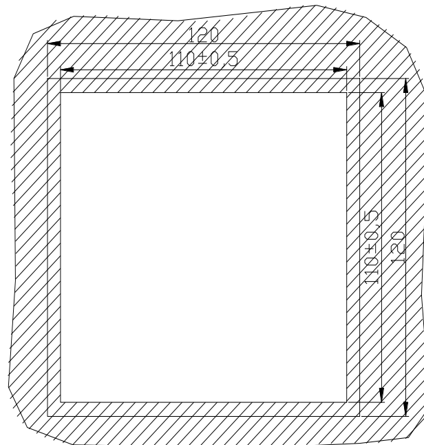
Рис. 2.2 Размеры вырубаемого окна в щите для установки щитового варианта указателя положения УП 2-Г с промежуточной рамкой
