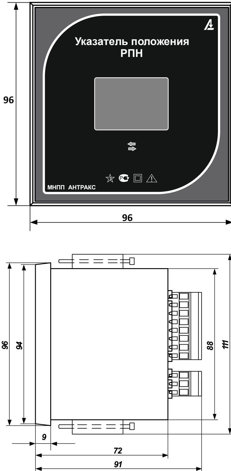
Рис. 1.1 Габаритные размеры щитового варианта указателя положения РПН УП 2-Г
