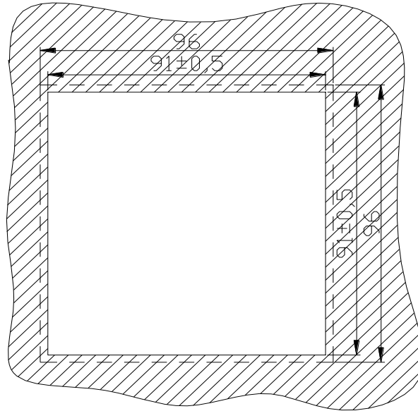
Рис. 2.1 Размеры вырубаемого окна в щите для установки щитового варианта указателя положения УП 2-Г
