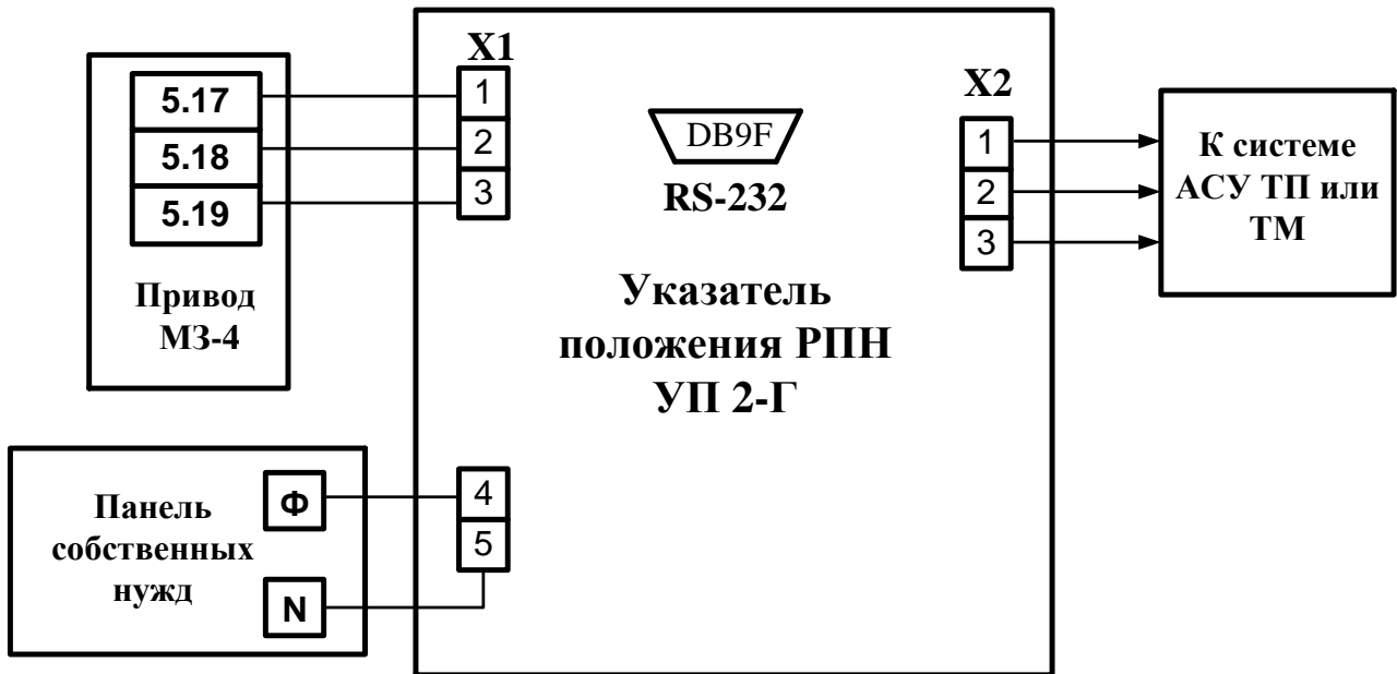
Рис. 4.1 Схема привязки УП 2-Г к приводу типа МЗ-2, МЗ-4.
