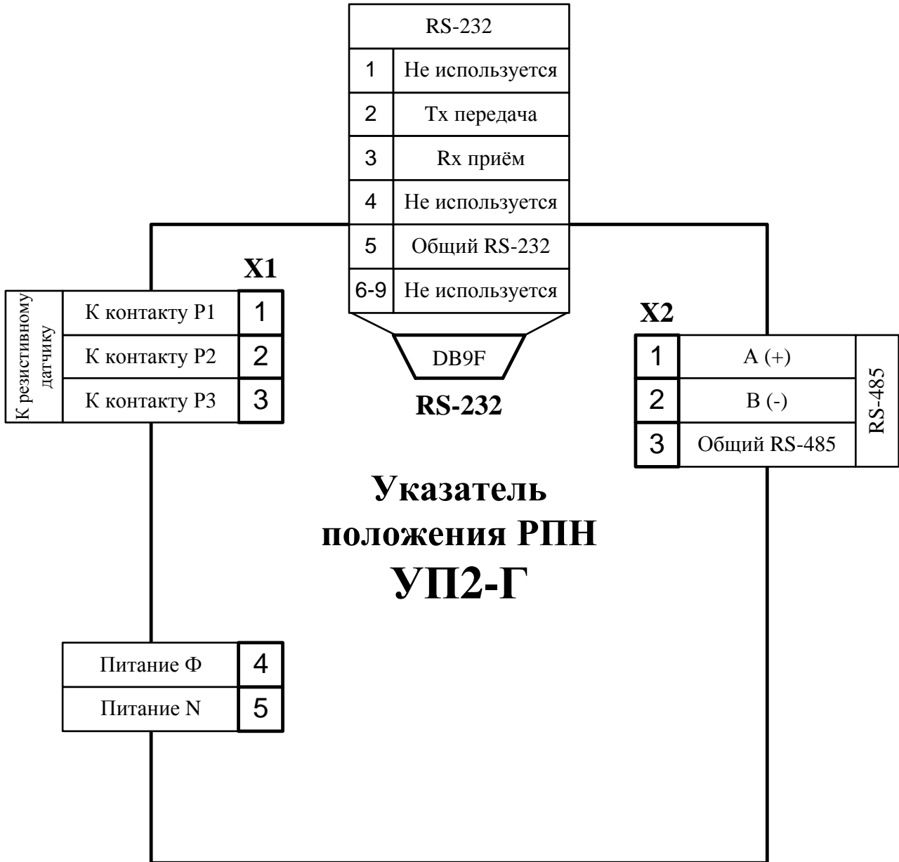
Рис. 3.1 Схема подключения УП 2-Г
