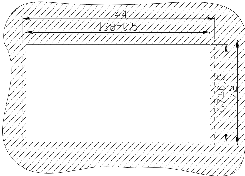
Рис. 2.1 Размеры вырубаемого окна в щите для установки щитового варианта указателя положения УП 23-Д
