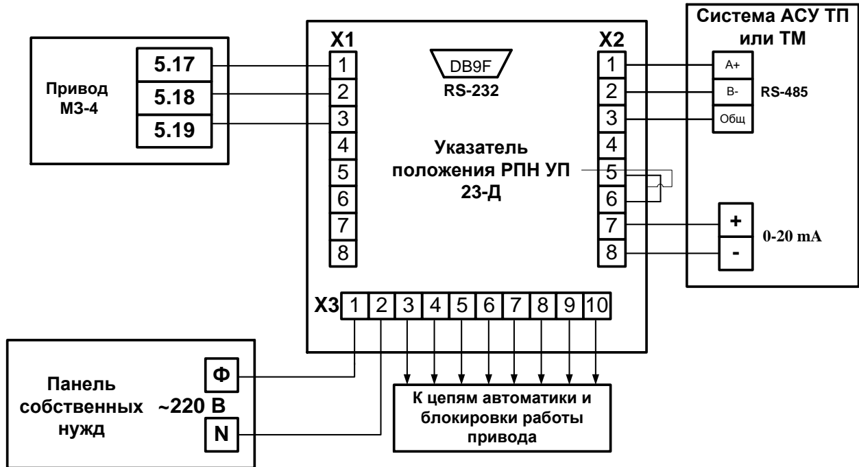
Рис. 4.1 Схема привязки УП 23-Д к приводу типа МZ-2, МZ-4.
