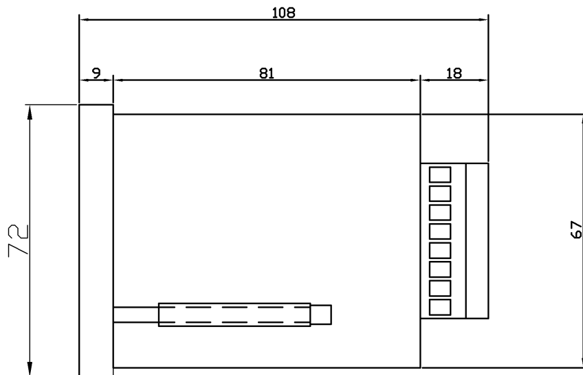
Рис. 1.1 Габаритные размеры щитового варианта указателя положения РПН УП 23-Д
