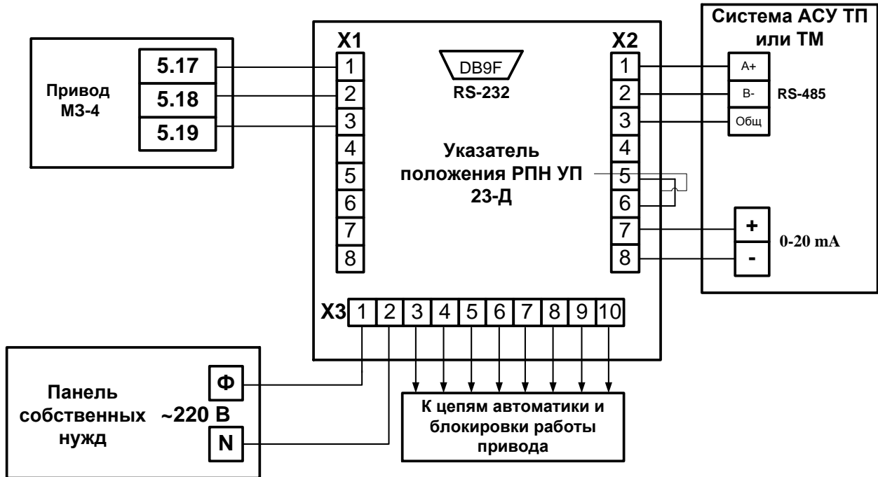
Рис. 4.1 Схема привязки УП 23-Д к приводу типа МЗ-2, МЗ-4.
