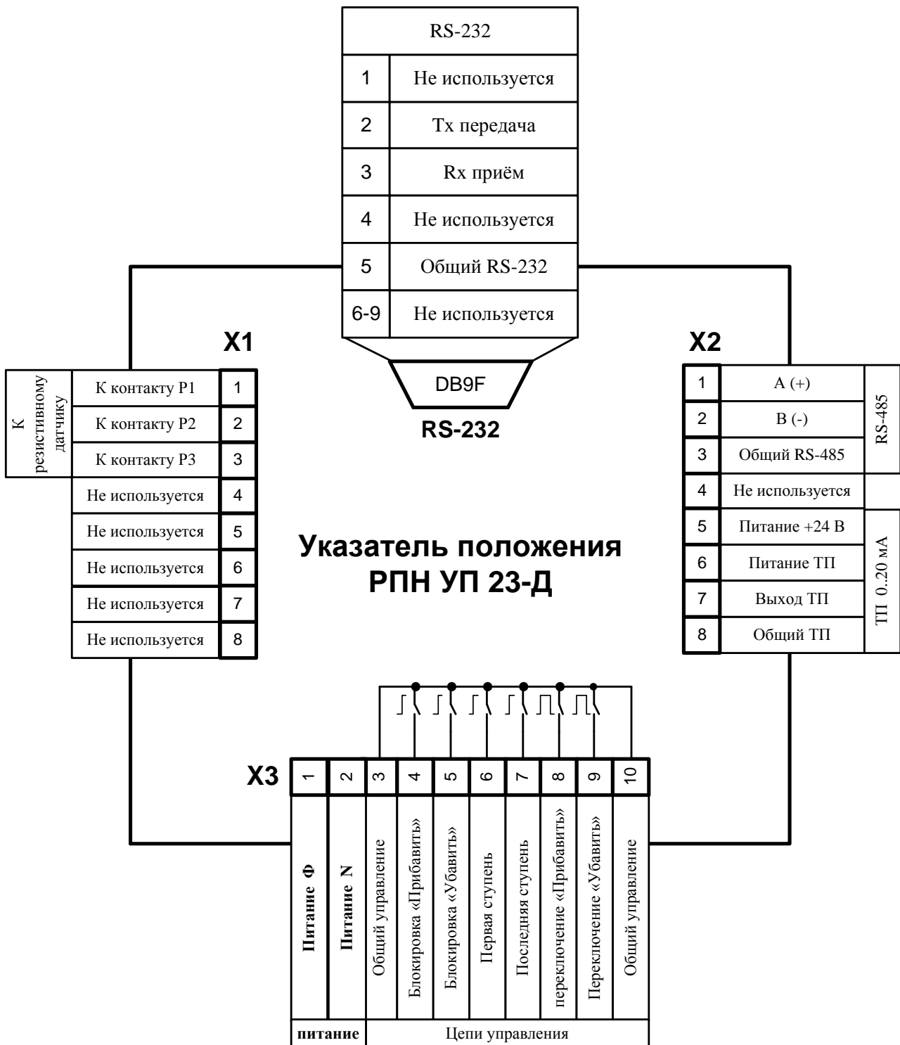
Рис. 3.1 Схема подключения УП 23-Д
