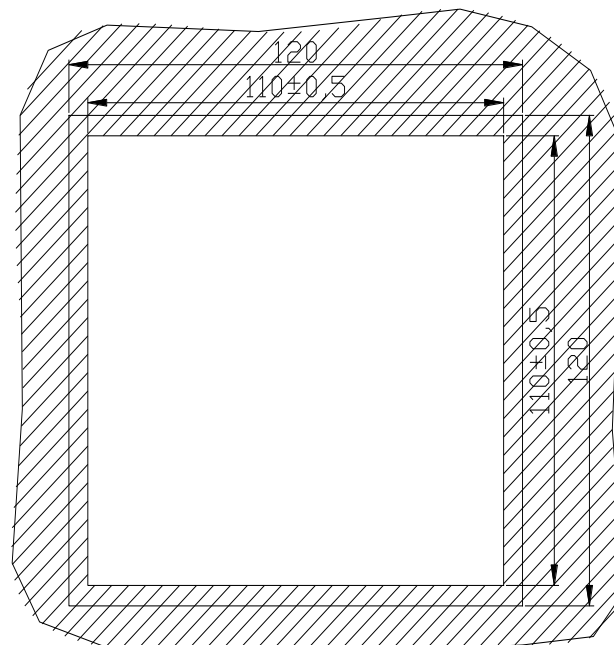
Рис. 2.2 Размеры вырубаемого окна в щите для установки щитового варианта указателя положения УП 23-Г с промежуточной рамкой
