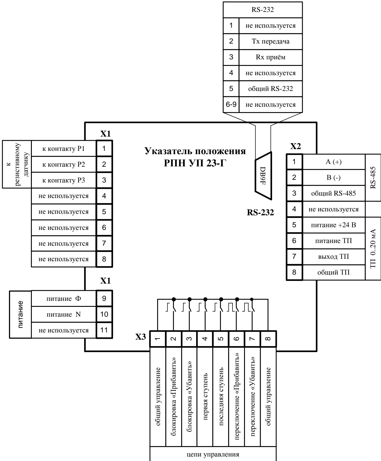
Рис. 3.1 Схема подключения УП 23-Г
