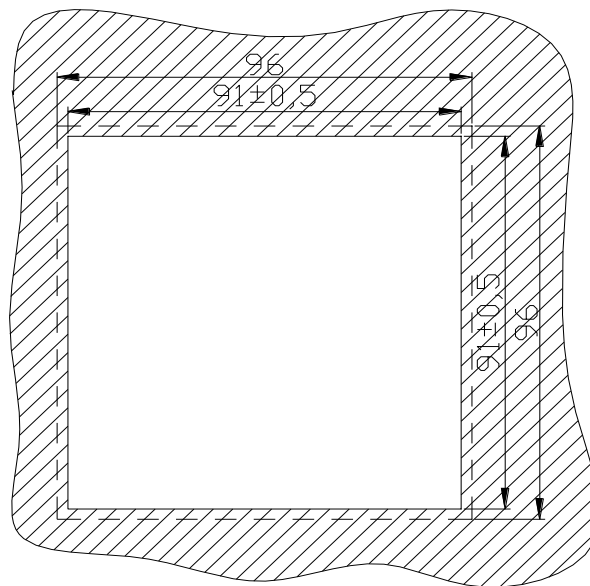
Рис. 2.1 Размеры вырубаемого окна в щите для установки щитового варианта указателя положения УП 23-Г
