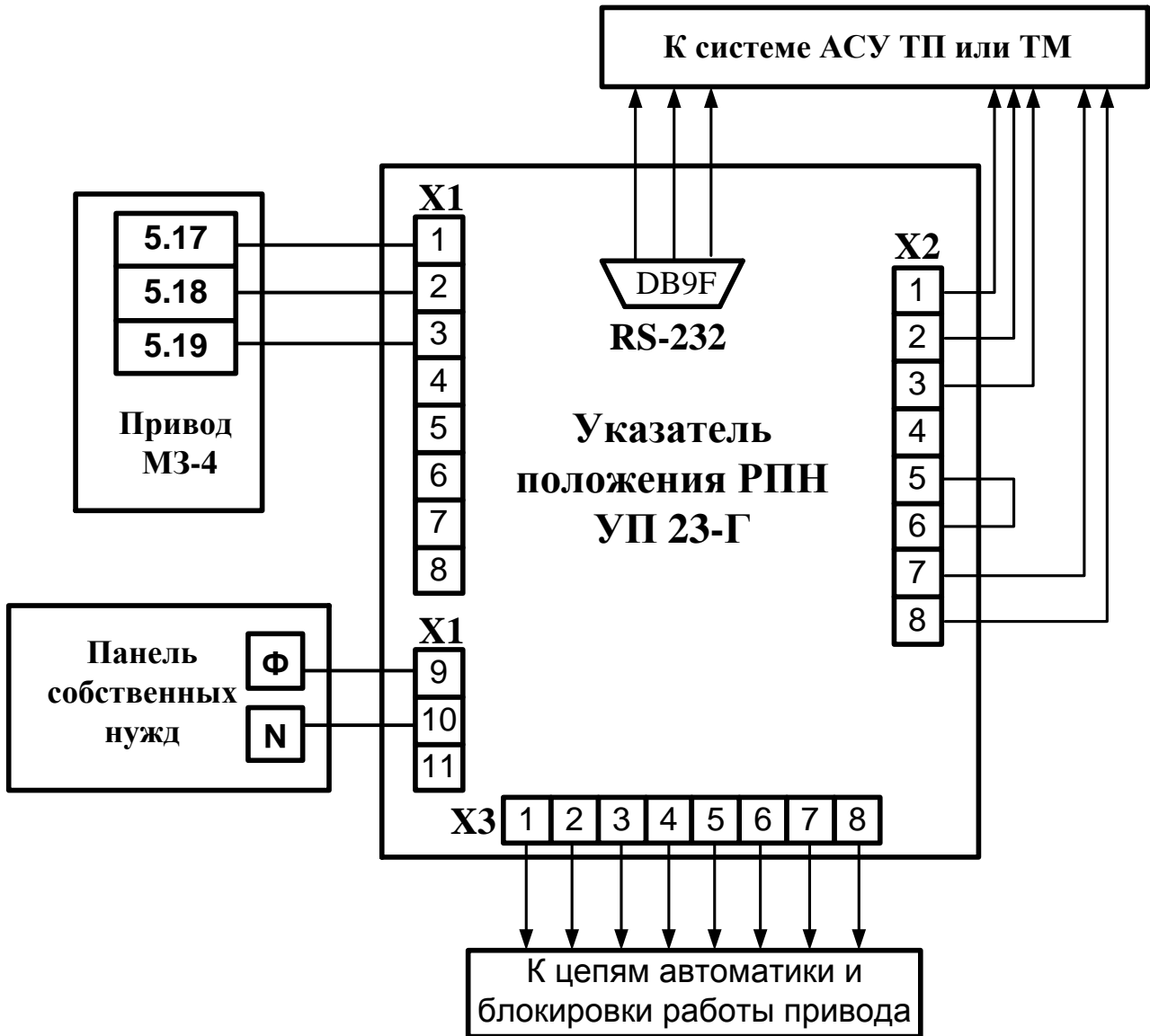
Рис. 4.1 Схема привязки УП 23-Г к приводу типа МЗ-2, МЗ-4.
