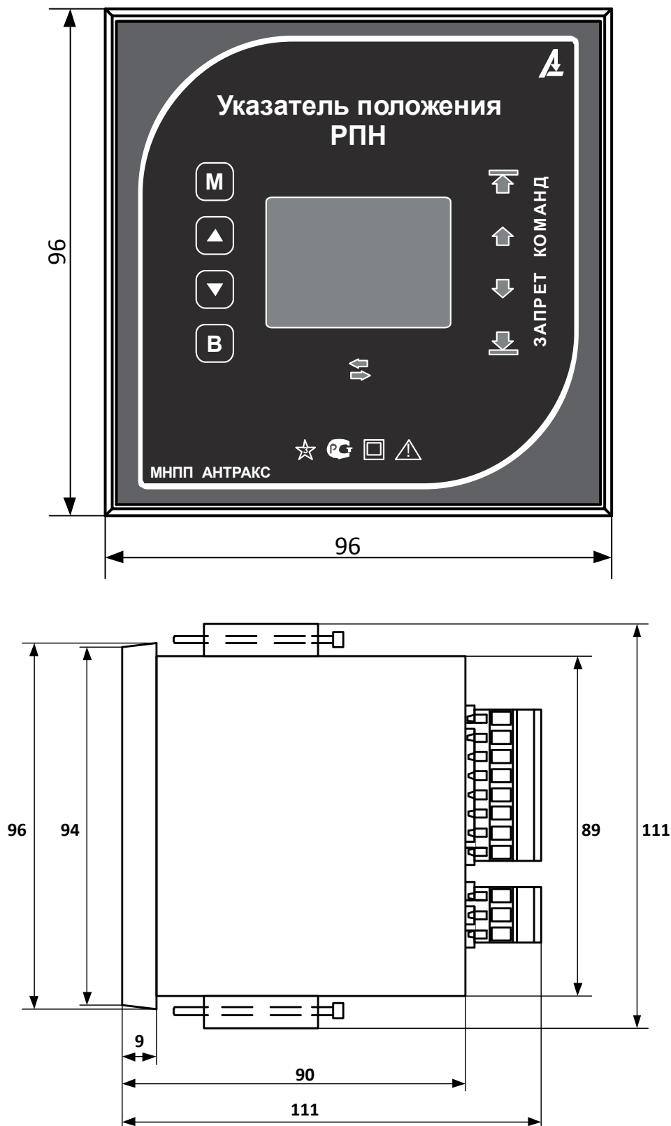
Рис. 1.1 Габаритные размеры щитового варианта указателя положения РПН УП 23-Г
