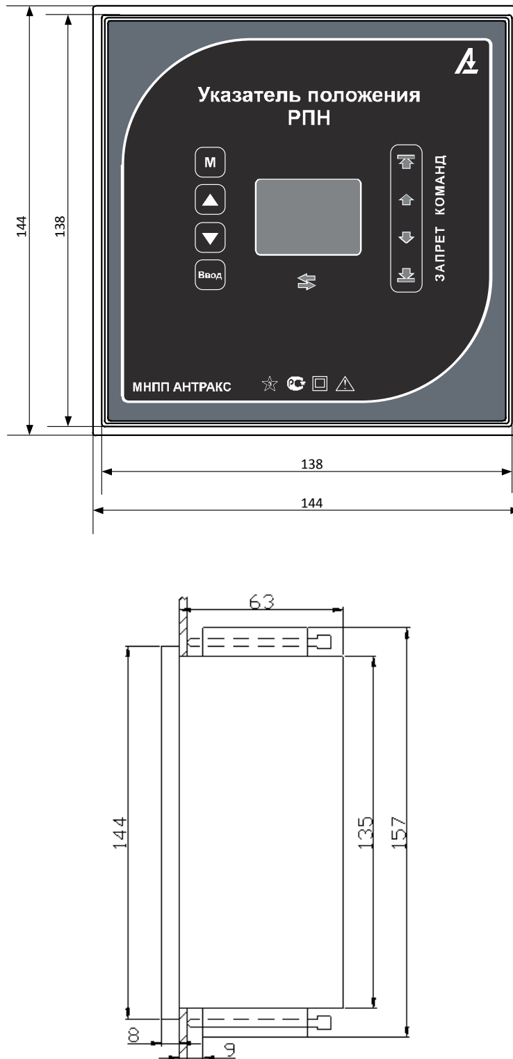
Рис. 1.1 Габаритные размеры настенного варианта указателя положения РПН УП 31-Б
