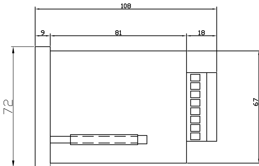
Рис. 1.1 Габаритные размеры настенного варианта указателя положения РПН УП 31-Д
