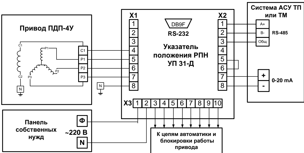
Рис. 4.1 Схемы привязки УП 31-Д к приводу типа ПДП-4У
