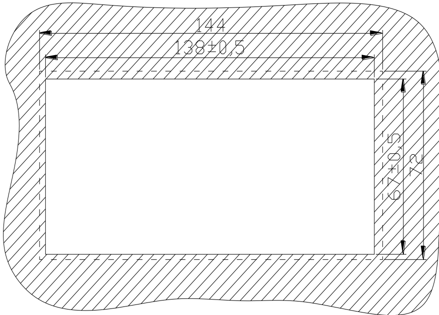
Рис. 2.1 Размеры вырубаемого окна в щите для установки щитового варианта указателя положения УП 31-Д
