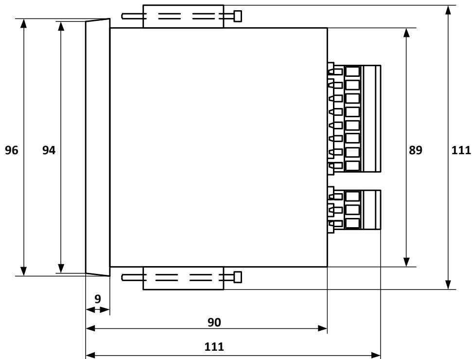
Рис. 1.1 Габаритные размеры настенного варианта указателя положения РПН УП 31-Г
